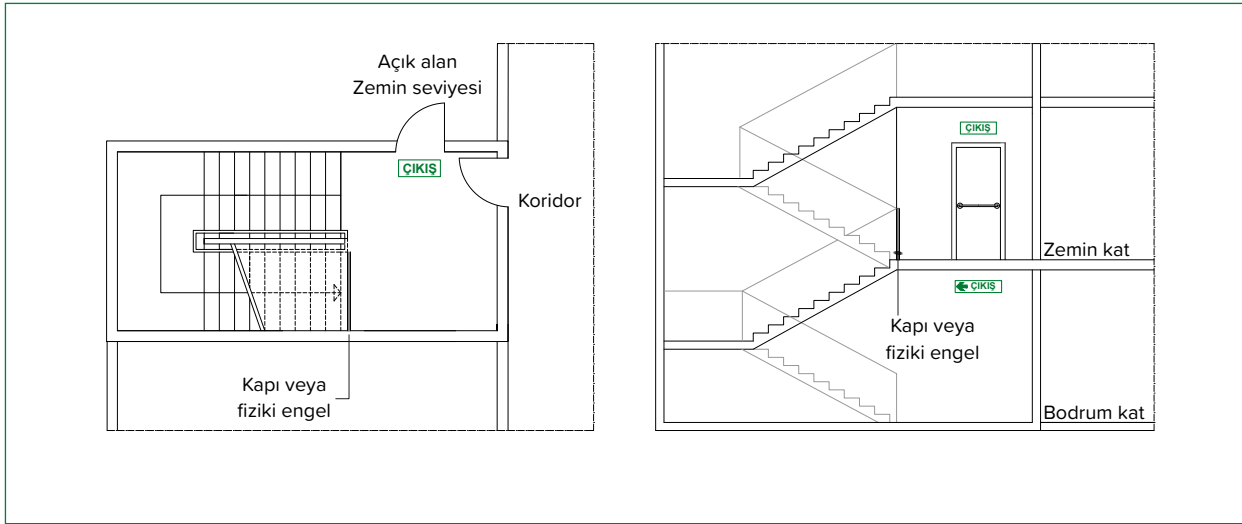
Şekil 46.2.b: Bodrum kat kaçış merdiveni
