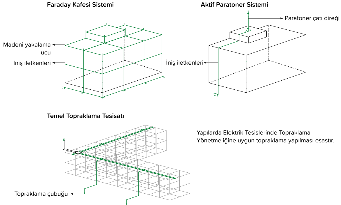
Şekil 64.1: Yıldırımdan korunma tesisatı
