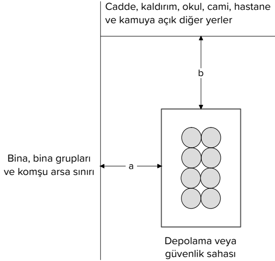
Şekil 106.12-13-14-15: Depo ve bina dışında LPG'nın tüplere doldurulmuş hâlde depolandığı mahal
