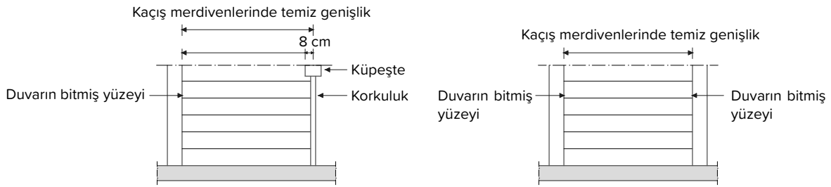
Şekil 148.1: Mevcut yapılarda kaçış merdivenlerinde genişlik
