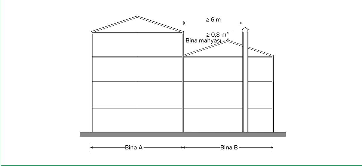
Şekil 58.2: Havalandırma bacası
