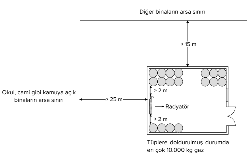
106.12-13 Özel olarak inşa edilmiş LPG dağıtım depoları
