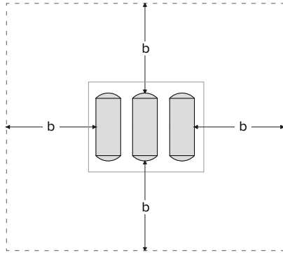
Şekil 119.3.b: Taşınabilir tanklarda koruma bölgesi
