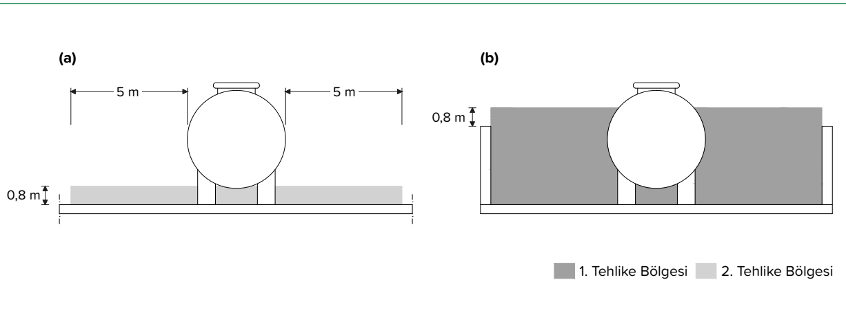
Şekil 119.4: Tehlike Bölgeleri
