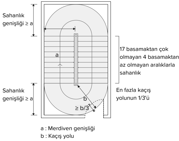
Şekil 41.3-4-5-6-7: Kaçış merdiveni özellikleri
