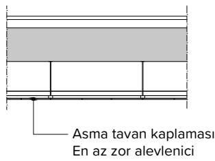
Şekil 26: Döşemeler
