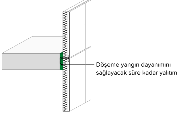
Şekil 27.3: Giydirme cephe sistemlerinde yangın güvenlik önlemleri
