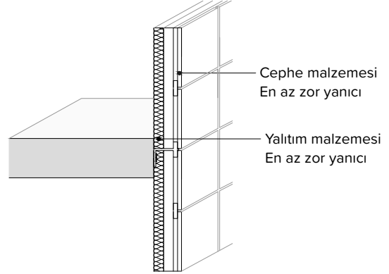
27.3.b Derzleri açık ve havalandırmalı giydirme cephe sistemli binalarda
