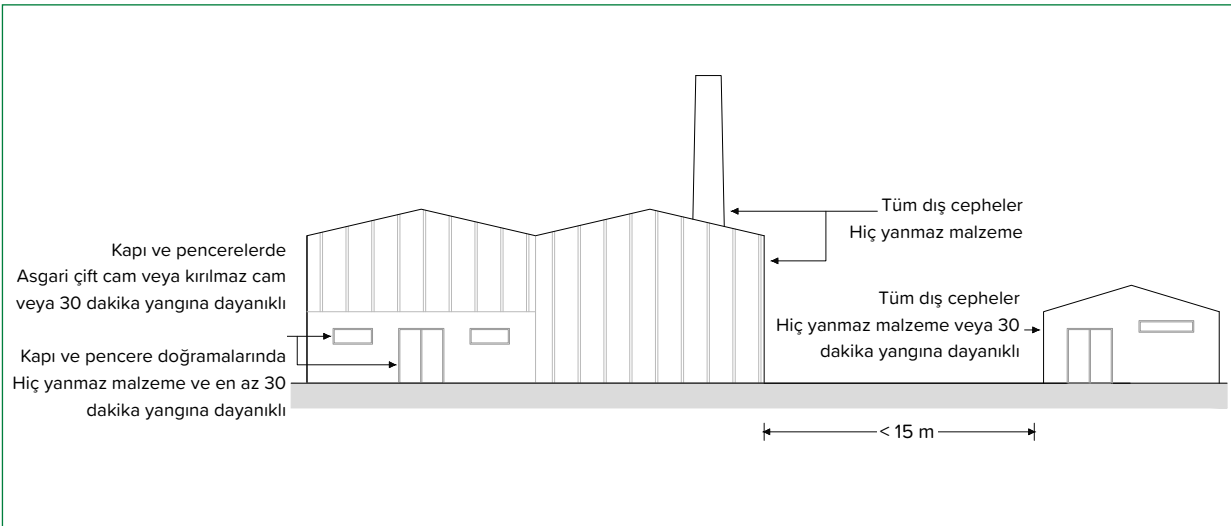
Şekil 27.4: Cephelerde yangın güvenlik önlemleri
